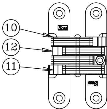
HINGE OPEN 180°
