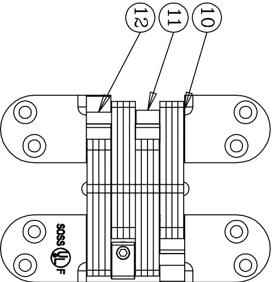
HINGE OPEN 180°
