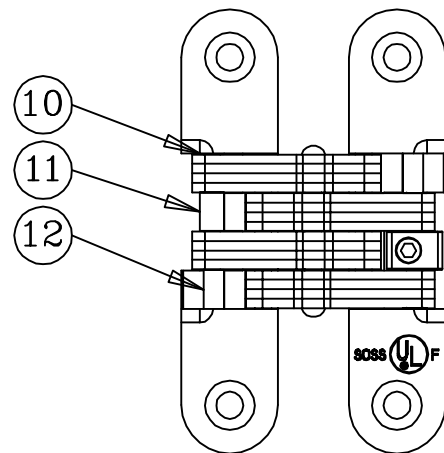
HINGE OPEN 180°
