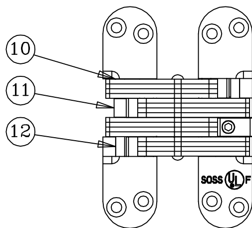
HINGE OPEN 180°
