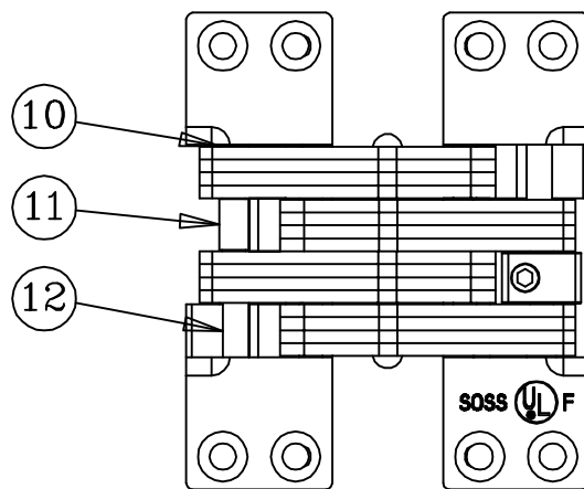
HINGE OPEN 180°
